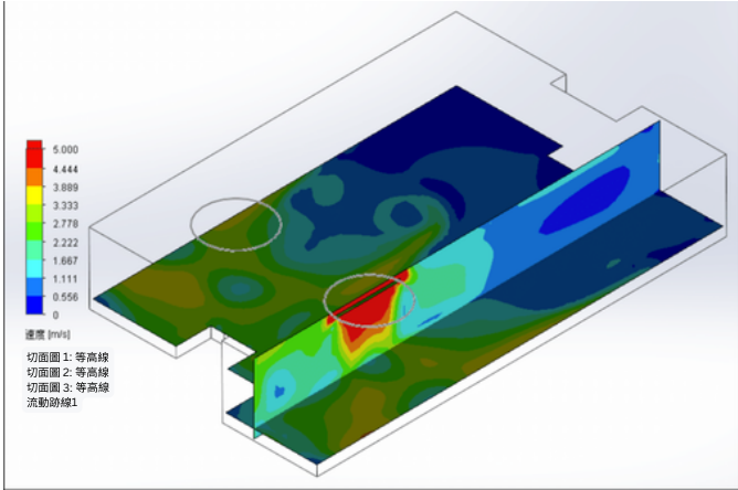
速度等值線圖 - 3 D 視圖
