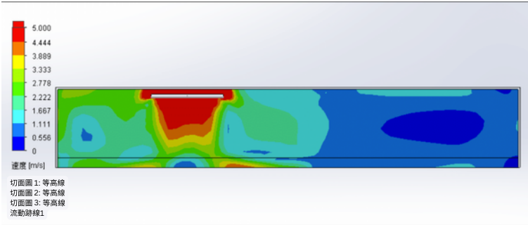
速度等值線圖 - 正視圖
