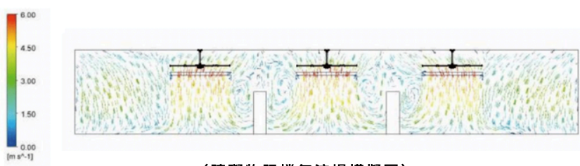
（障礙物阻擋氣流場模擬圖）
