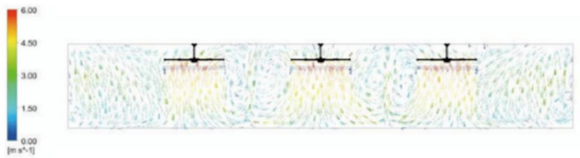
（多台氣流場模擬圖）
