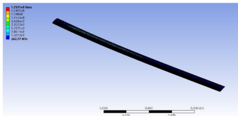
圖二：風扇葉片應力圖
